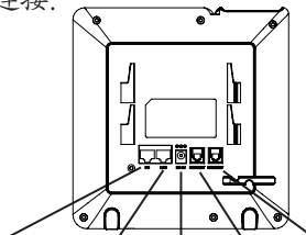
PC端口 网络连接端口 5V电源 耳机 手柄
