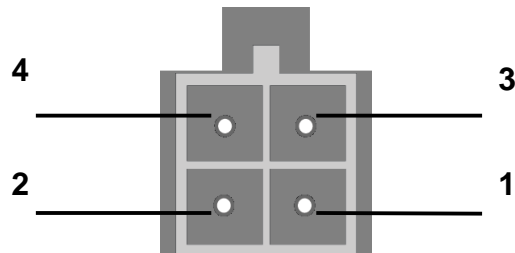
Рис. 3.4. Разъем питания
